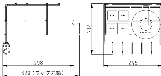
製品寸法
